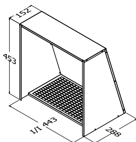
322. CH-350 CH-350 CP Chairmans Hat 350ø
